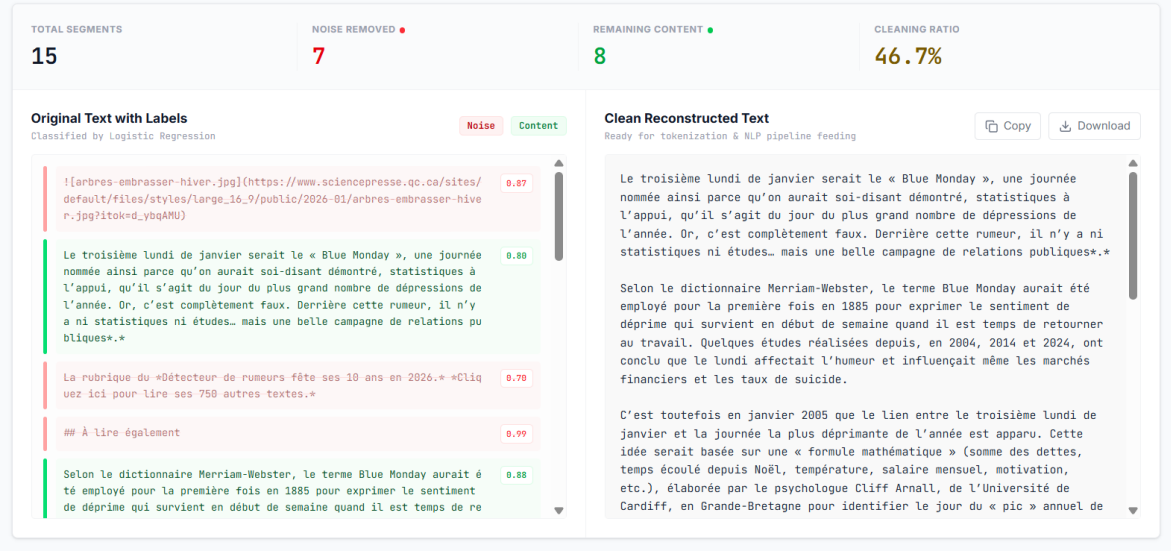
Fig. 3.3 : Tableau de bord de résultats utilisé pour synthétiser les performances expérimentales de NoiseCleaner.
