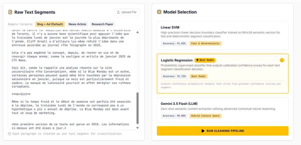
Fig. 3.2 : Interface de sélection du modèle utilisée pour comparer les classifieurs supervisés de NoiseCleaner.
