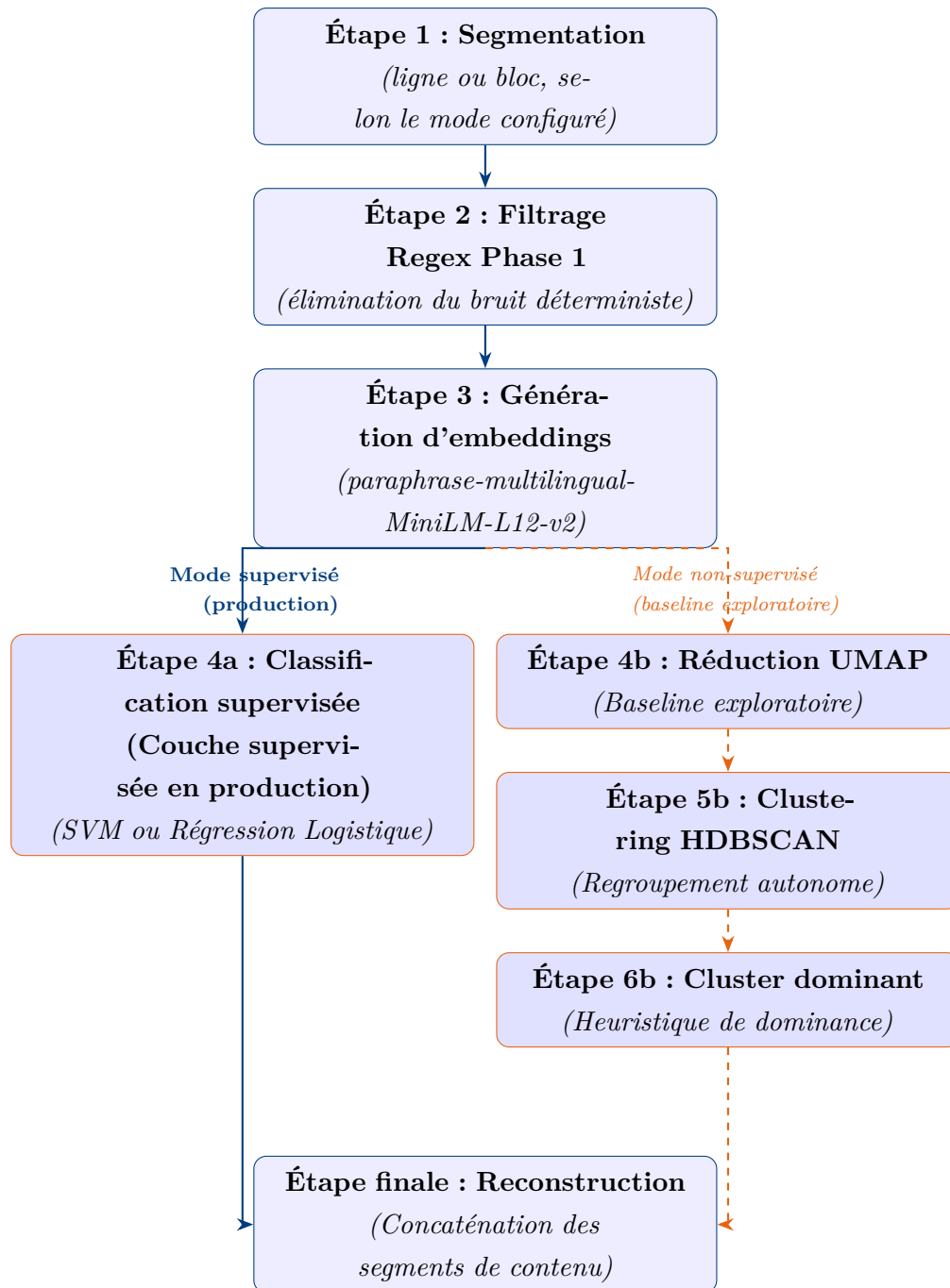
Fig. 2.9 : Décomposition méthodologique du pipeline NoiseCleaner en mode supervisé hybride et en baseline exploratoire non-supervisée.
