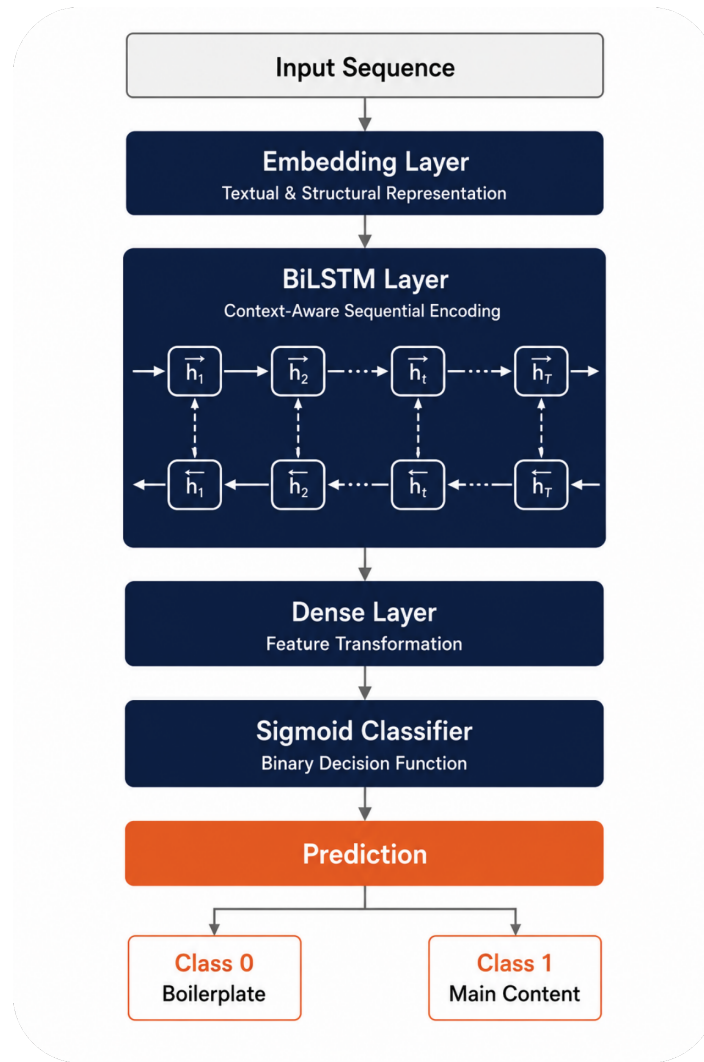
Fig. 1.5 : Architecture neuronale de BoilerNet basée sur une couche BiLSTM suivie d'un classificateur Sigmoid pour la détection du contenu principal et du bruit de type boilerplate.
