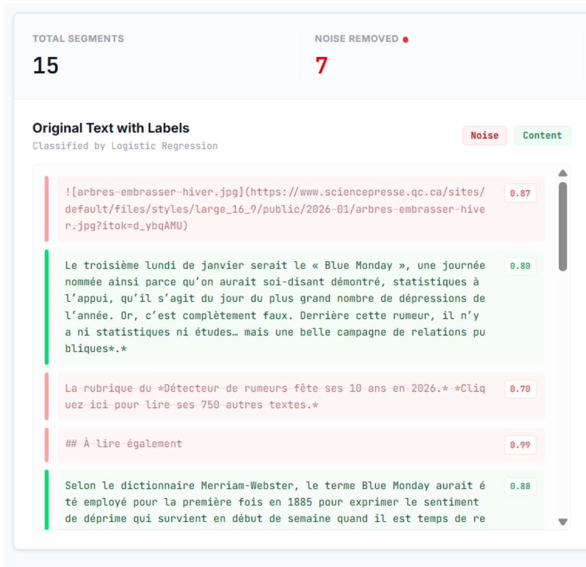
Fig. 3.4 : Visualisation de la classification segmentaire entre contenu utile et bruit.
